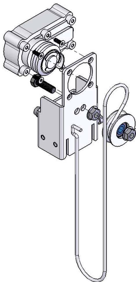
L-opening door
