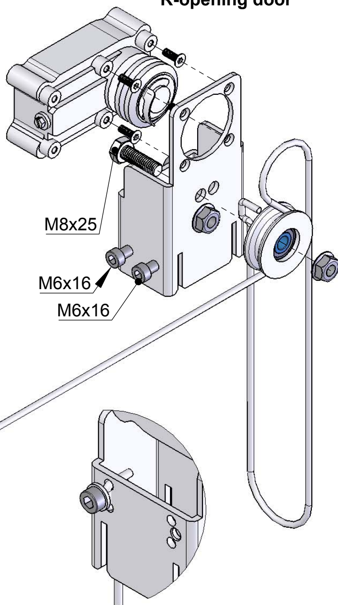
R-opening door
