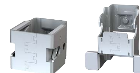
COLLIER SUPÉRIEUR RAPID FIX Le panneau est verrouillé par la fonction clic intégrée. Démontable rapidement à l'aide d'un outil.
