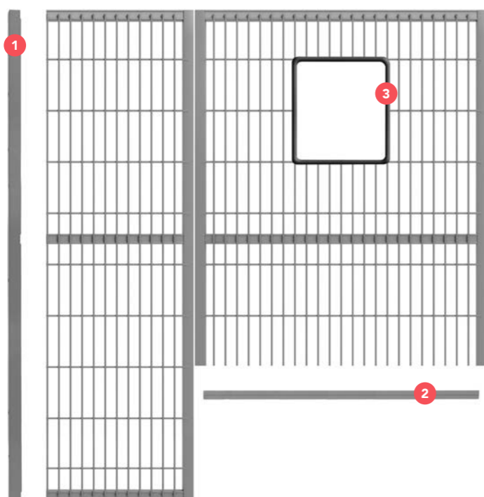
KIT POUR DOUBLAGE PETG Ce kit permet de fixer une plaque de polycarbonate sur le panneau grillagé pour empêcher les projections et les éclats.
