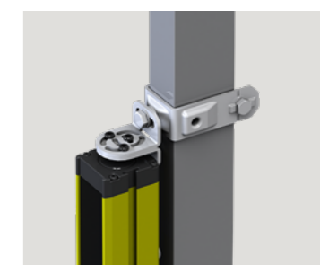
SUPPORT DE FAISCEAU LUMINEUX Fixez différents types de faisceaux lumineux directement sur les poteaux Troax à l'aide du support réglable Smart Fix.
