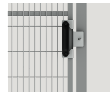
SERRURE MAGNÉTIQUE Poignée en plastique solide montée sur la butée de porte.
