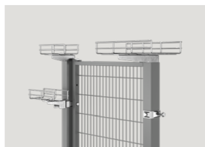
CHEMIN DE CÂBLES ET SUPPORTS Fixation facile des consoles aux poteaux ou support Smart Fix pour chemins de câbles de 100mm ou 200mm de largeur.
