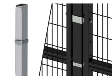
SMART SPLICE Support qui s'intègre dans les tubes 60 x 40 pour réhausser les poteaux.
