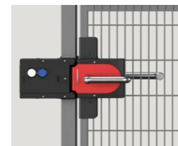
EUCHNER MGB, MGB-PN Support compatible avec tous les modèles sur tous les types de portes.
