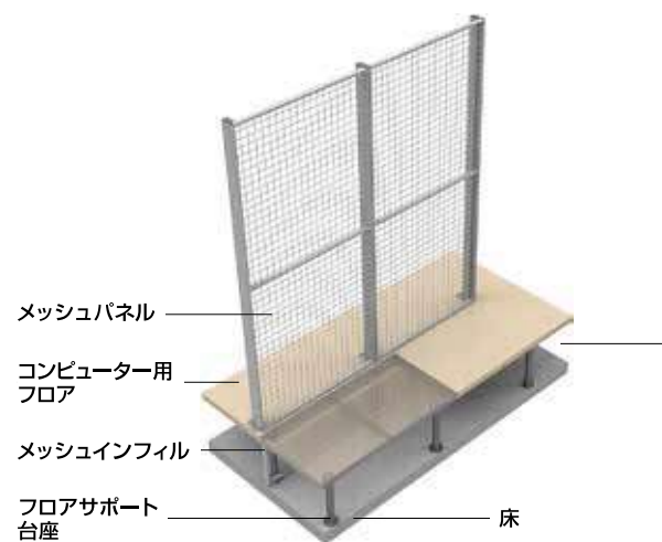
床とコンピューター用フロアの間に敷いたメッシュインフィルの例。
