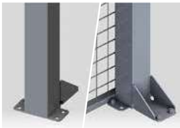
7 ポスト 80×80
